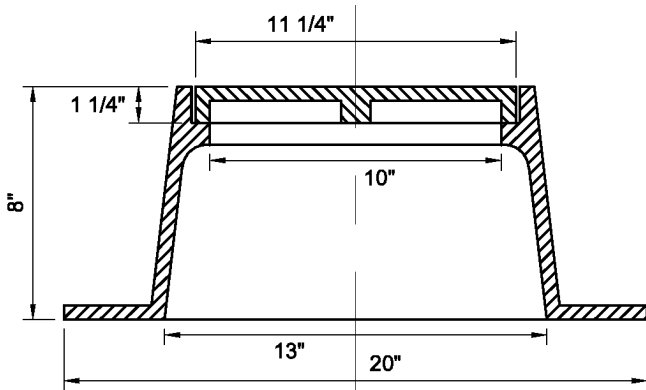
FRAME & LID
